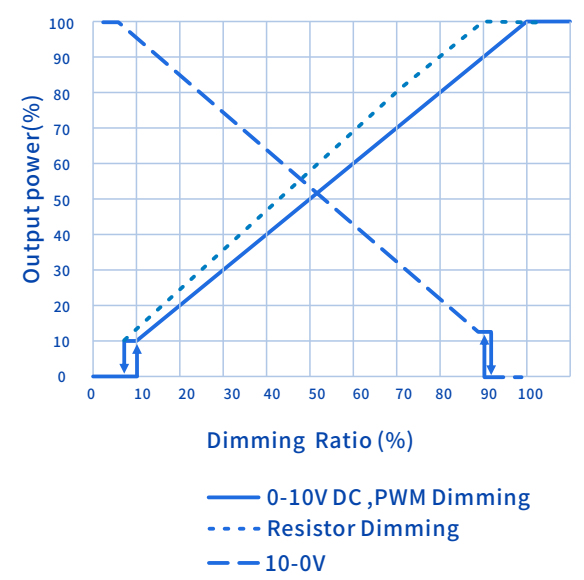
输出功率Vs.调光信号
